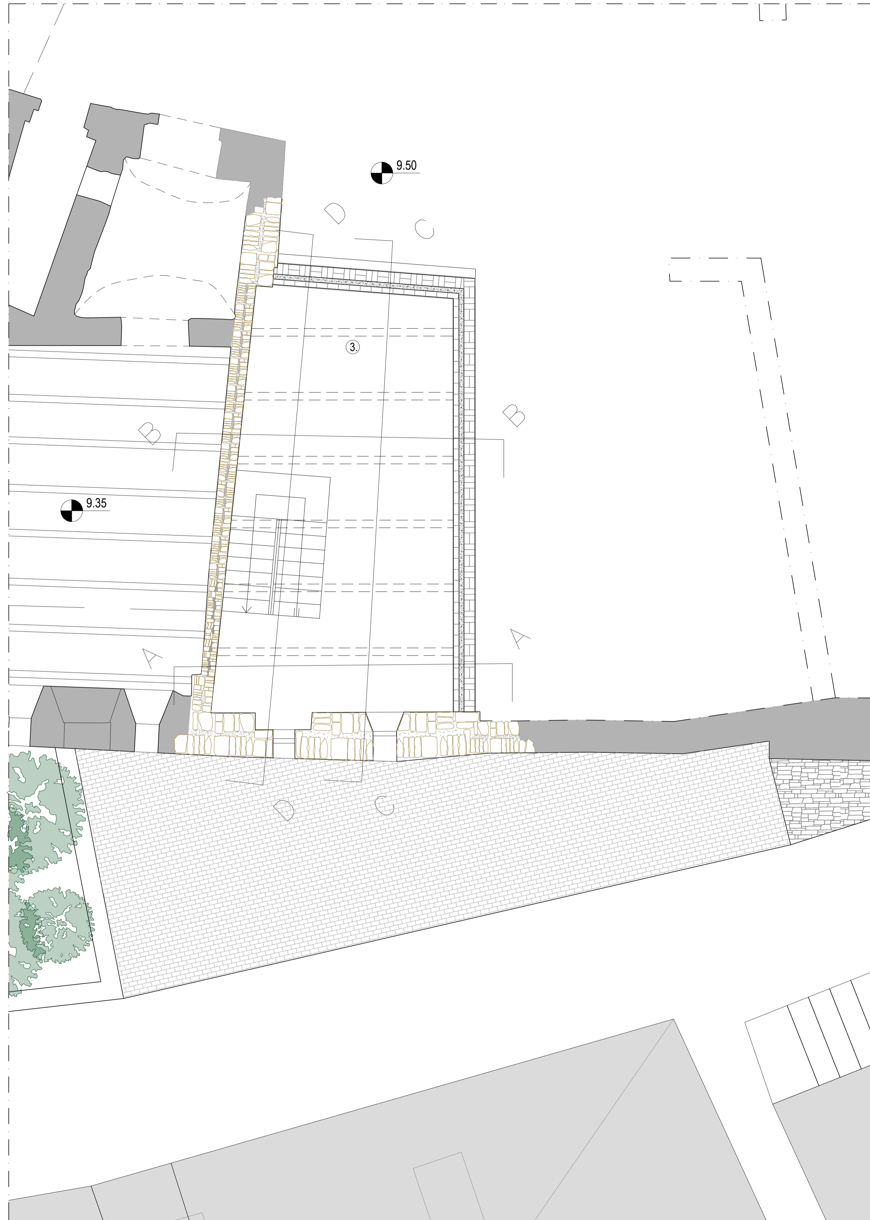
Pianta quota +12m
