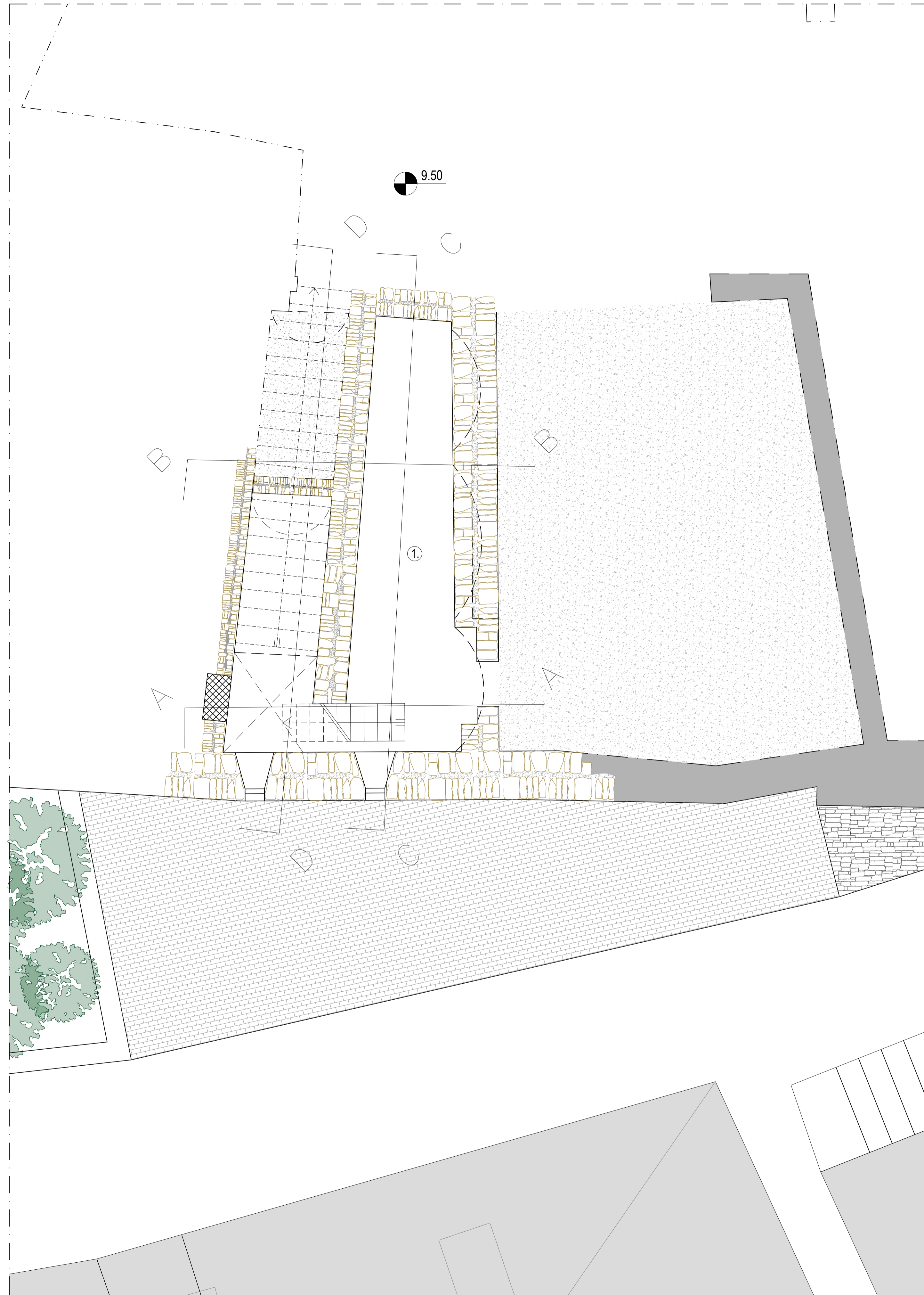
Pianta quota +6m
