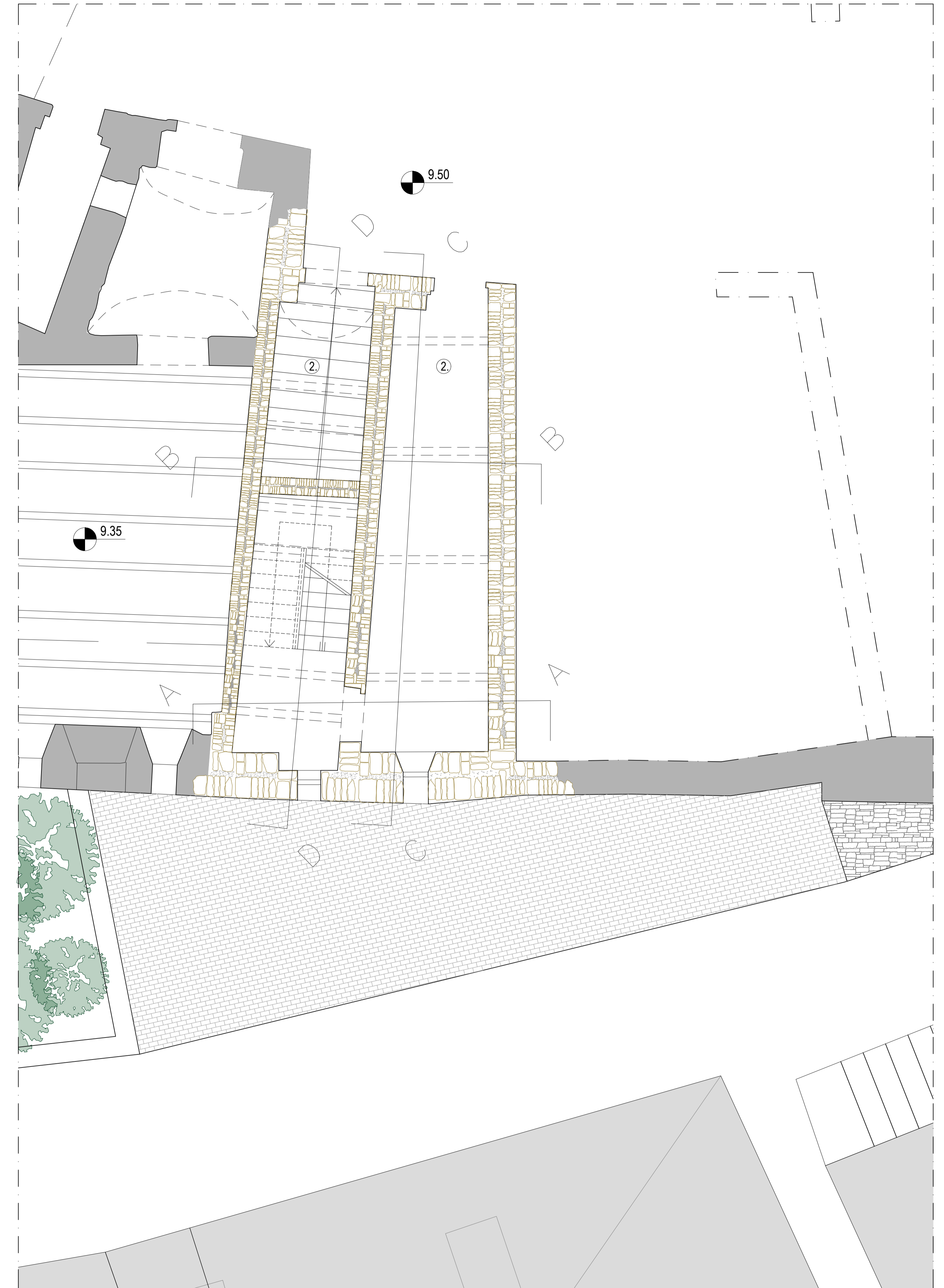
Pianta quota +10m
