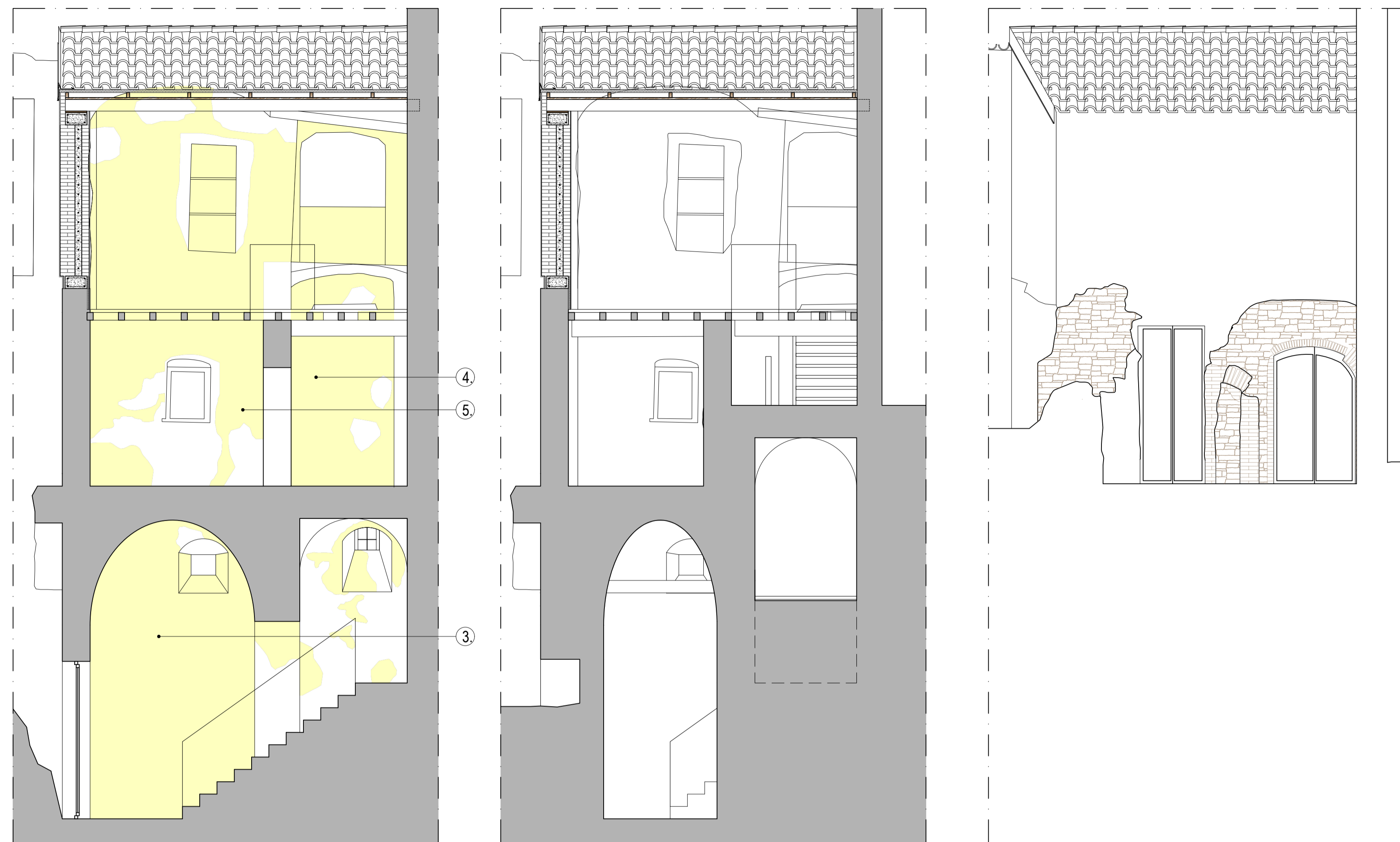
Sezione A-A
