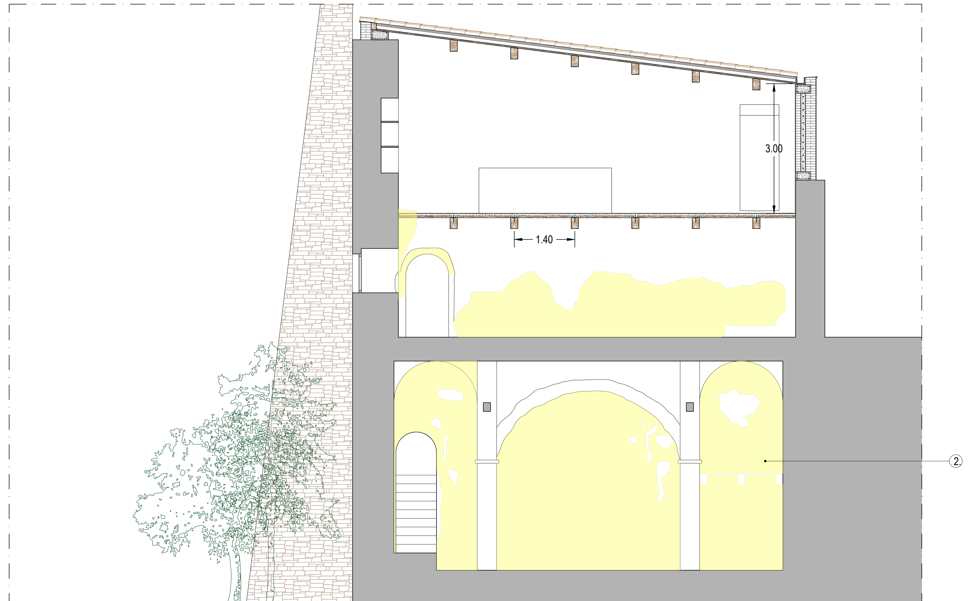
Sezione C-C
