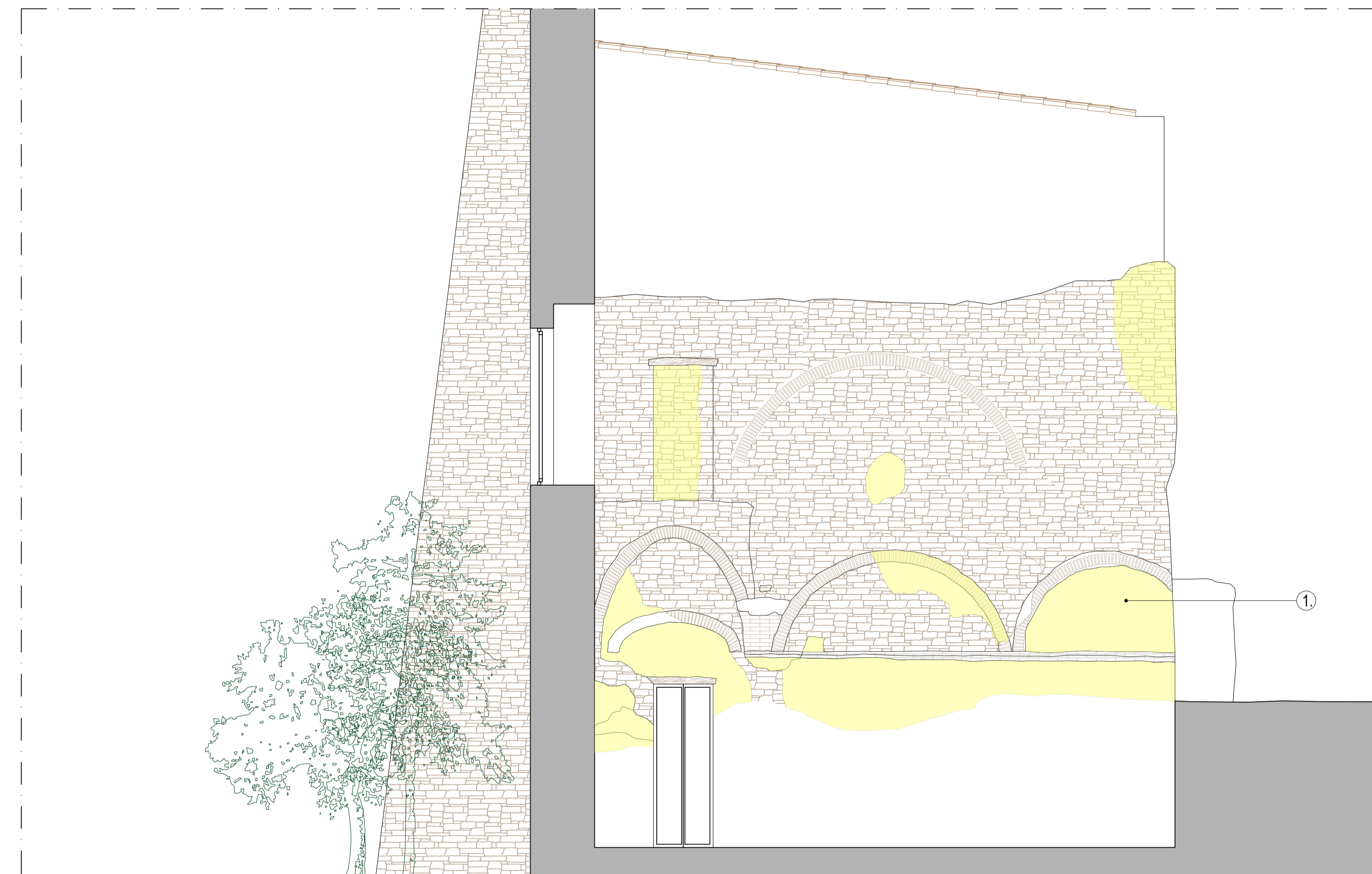
Prospetto sud-est
